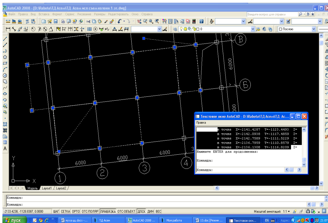
5 Сурет – AutoCAD бағдарламасынан геодезиялық бөлу координаттарын алу
