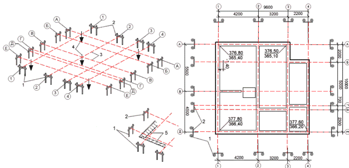
4 Сурет – Құрылыстың негізгі өстерін бөлу жұмысы
